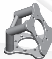
ISX15-DC60 Соединительный модуль с углом наклона 60 градусов
